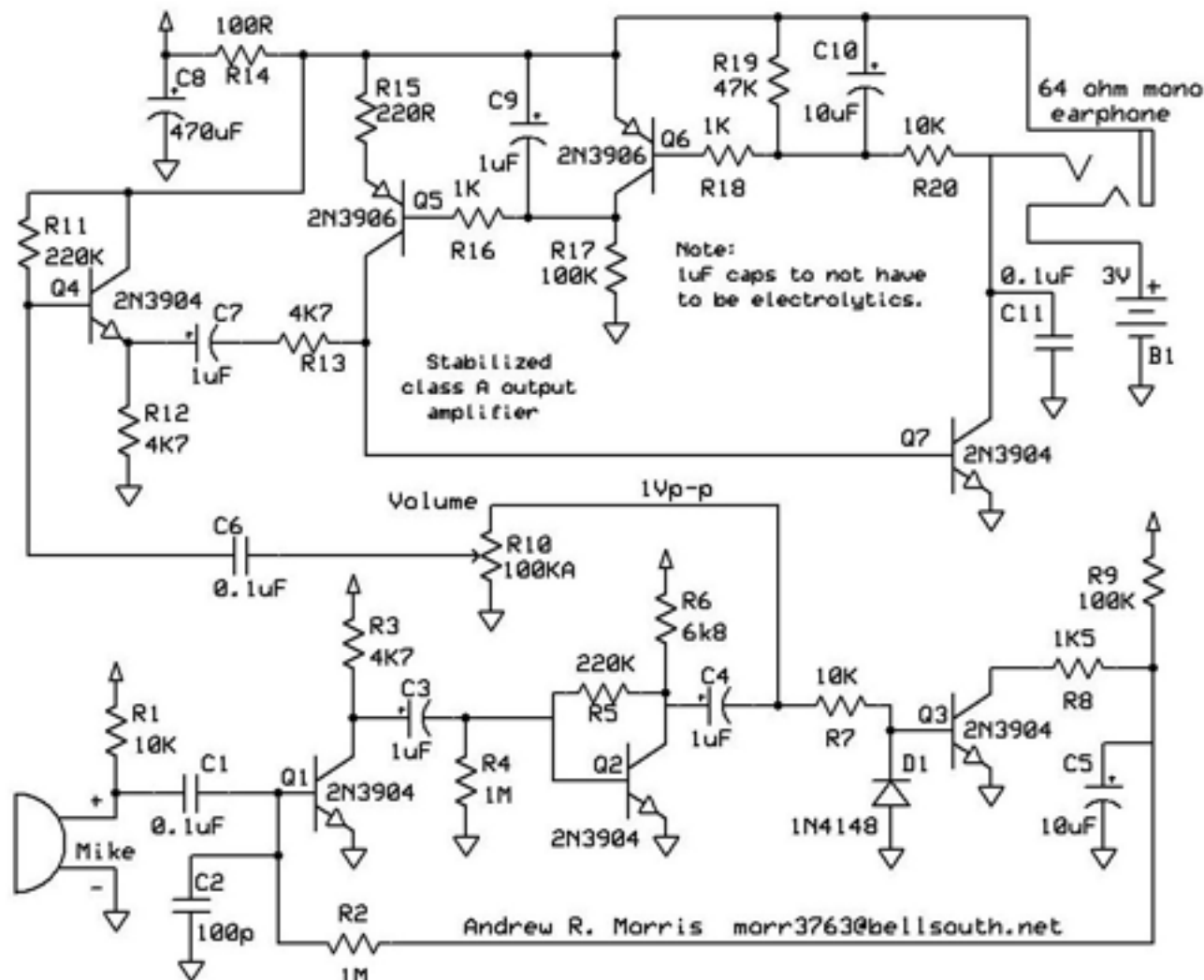
Listen Amplifier (3 Volt Version)
